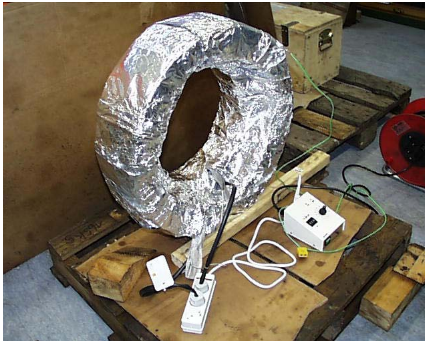
Überprüfung von Hydraulikmuttern im Kundenauftrag zur Ermittlung von Drucksteigerungen bis 100° C
